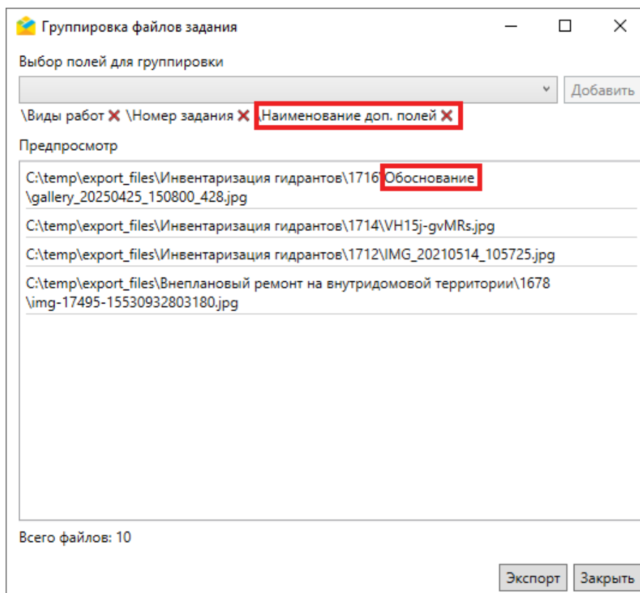
Рис. 2.147: Путь экспорта файла, прикрепленного к файловому полю задания
