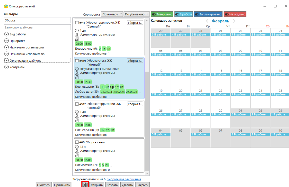
Рис. 2.218: Выбор расписания для экспорта
