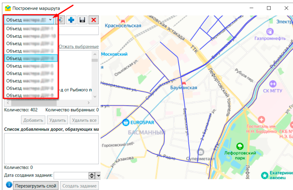
Рис. 2.200: Выбор маршрута из заранее сохраненного шаблона
