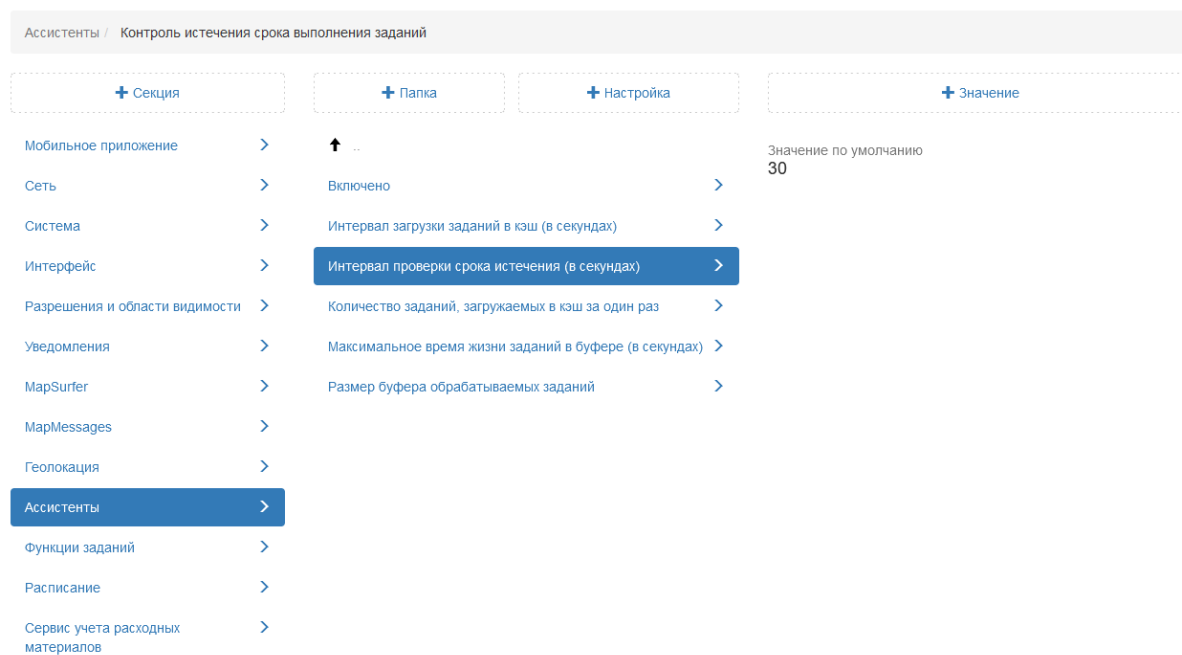
Рис. 2.233: Интервал проверки истечения срока
