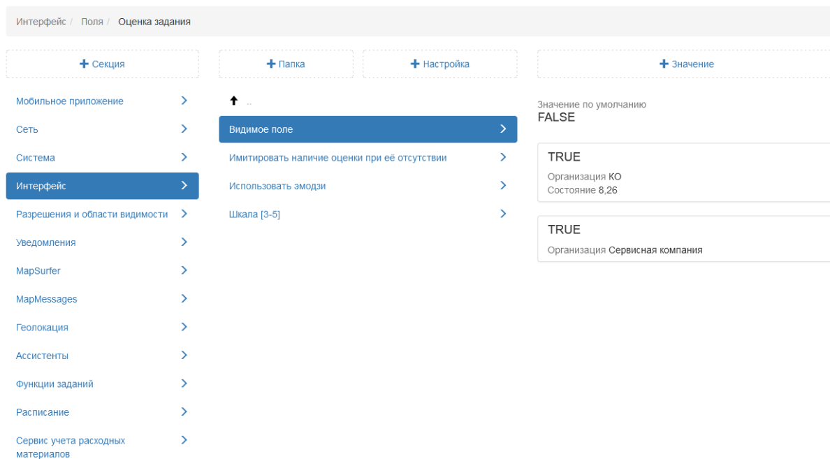
Рис. 2.155: Настройка видимости оценки
