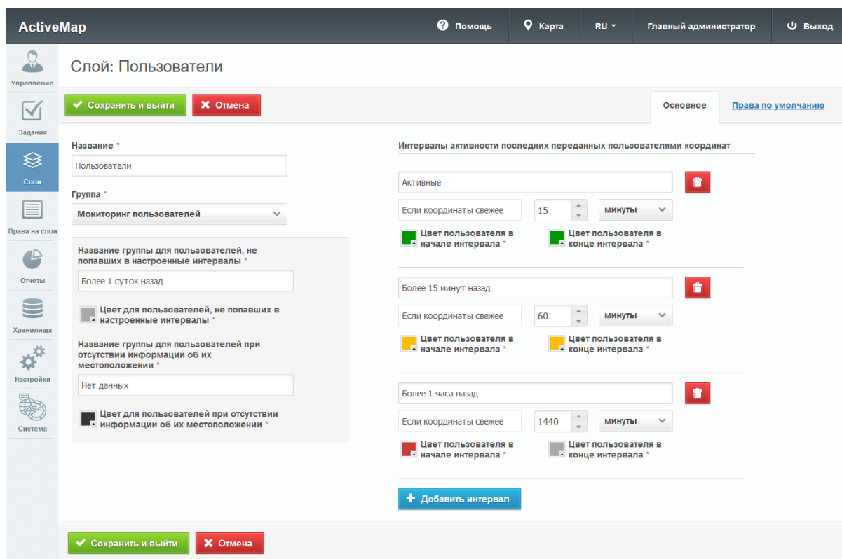
Рис. 2.63: Редактирование отображения системного слоя «Пользователи»
