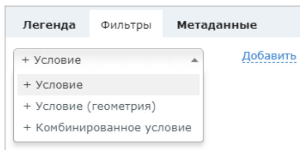
Рис. 2.18: Виды фильтров
